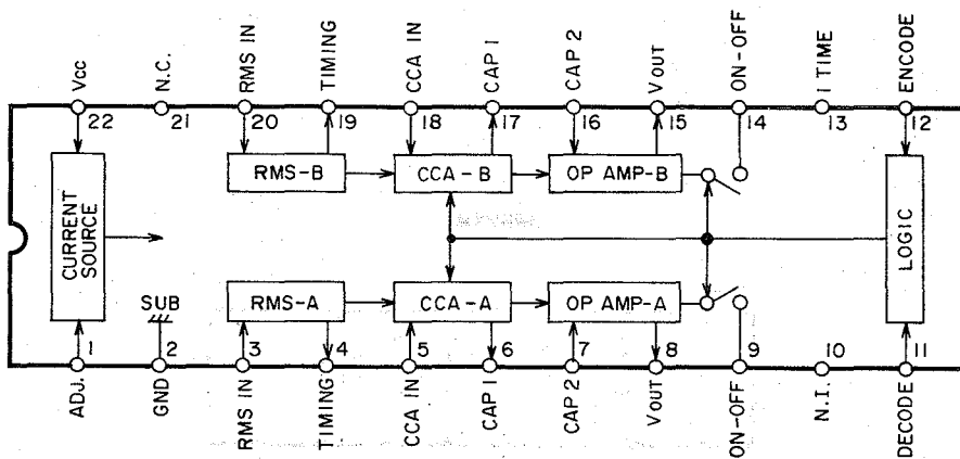
AN6291
