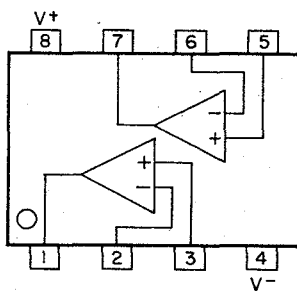
M5220P
